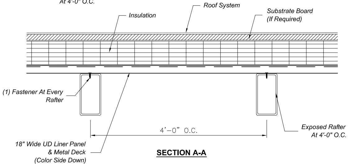
TYP UD LINER APPLICATION
